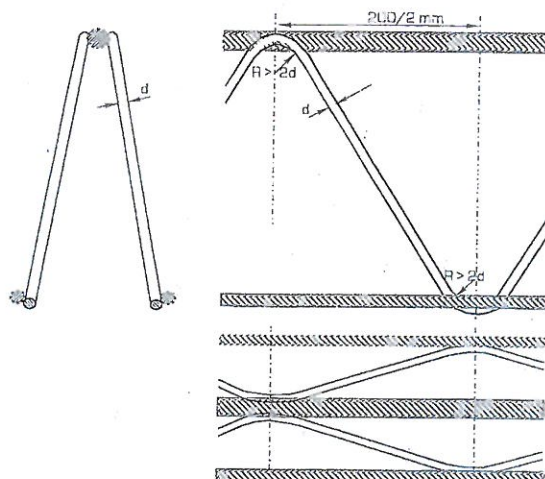
FILIGRAN E-Träger
