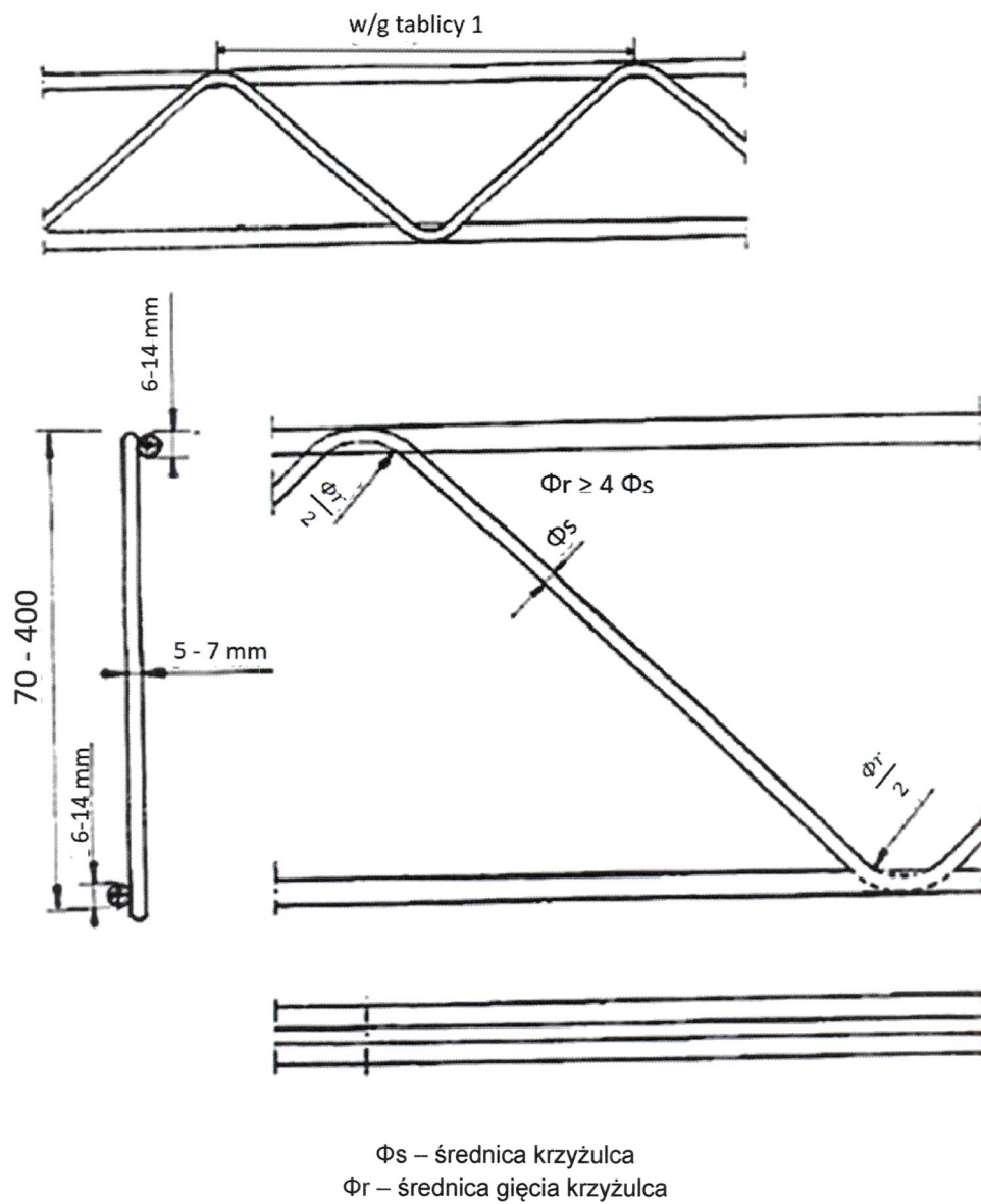
Rys. A8. Kratownica stalowa FILIGRAN EH
