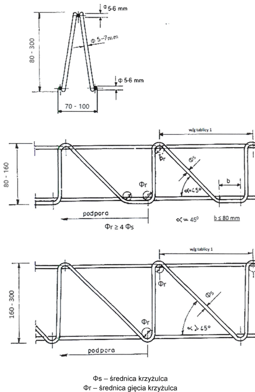
Rys. A4. Kratownica stalowa FILIGRAN EQ
