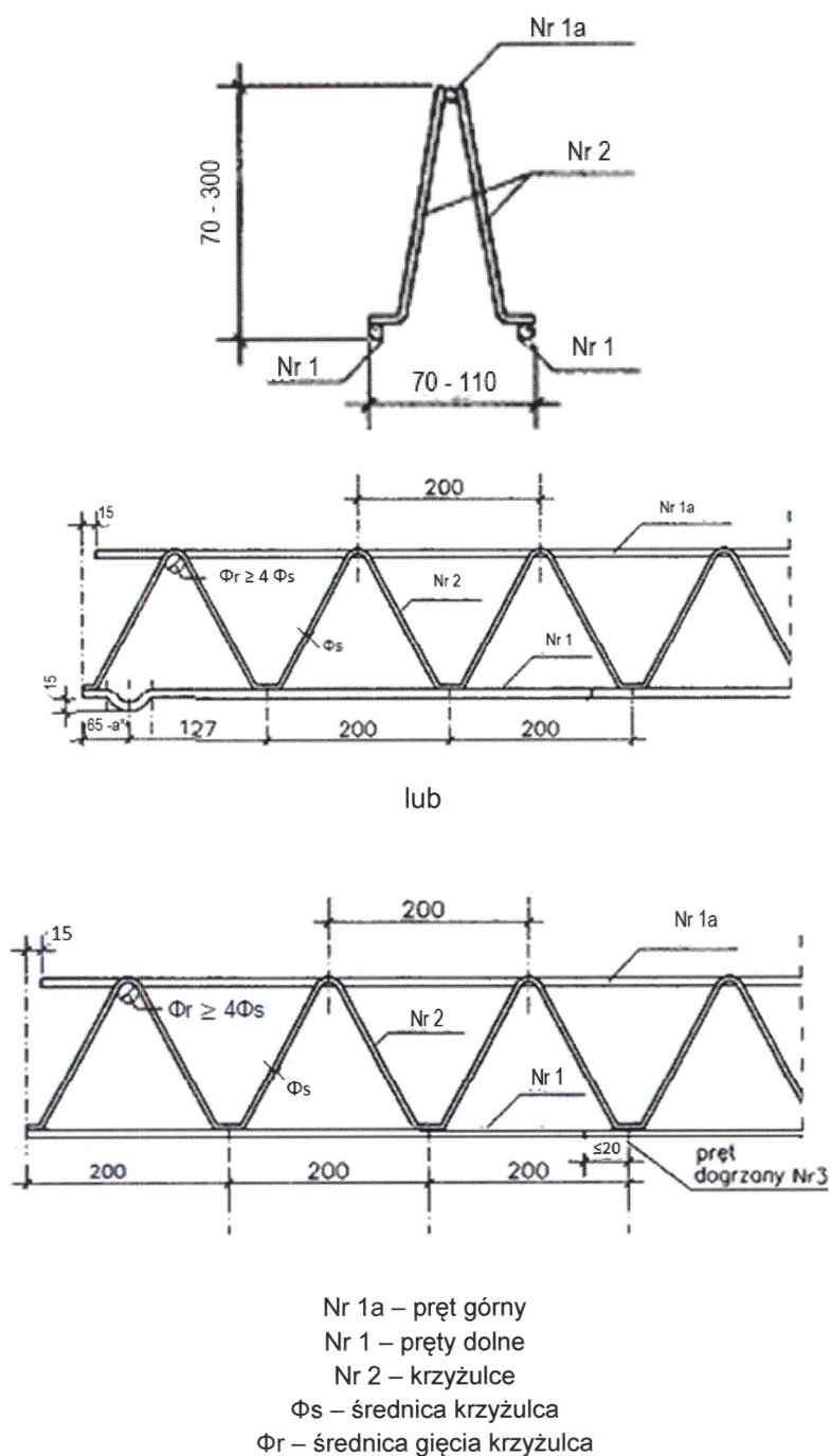
Rys. A3. Kratownica FILIGRAN EK
